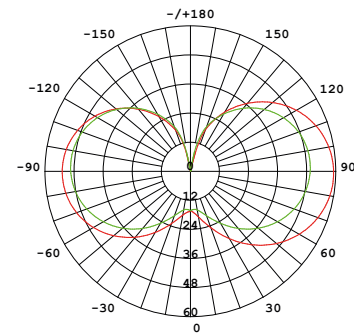
CURVA FOTOMETRICA
